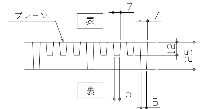
FRPグレーチング断面図
