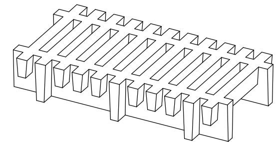
F R P グレーチング詳細
