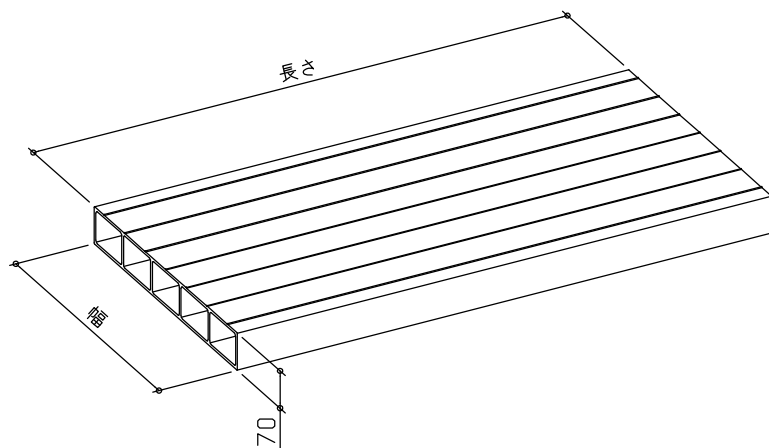
グラスファイバーデッキ詳細図
