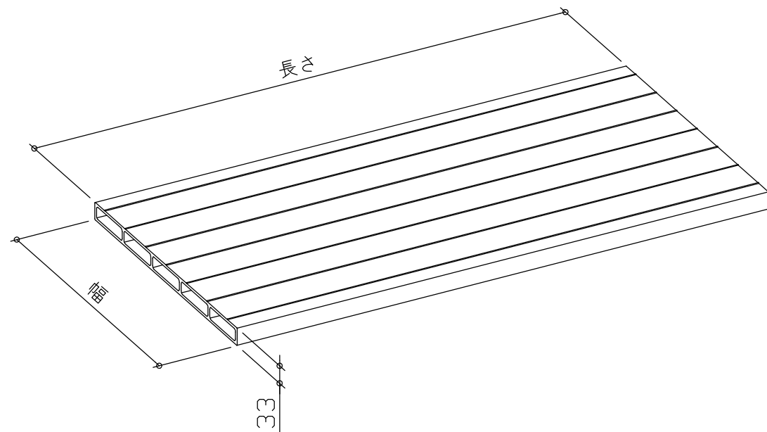
グラスファイバーデッキ詳細図
