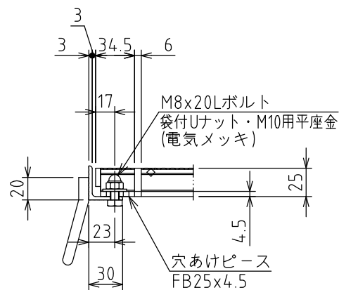
ボルト固定部詳細図
