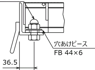
ボルト固定部詳細
