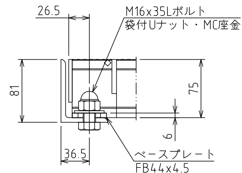
ボルト固定部詳細図
