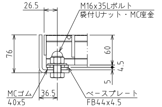
ボルト固定部詳細図
