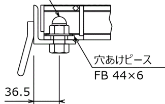
ボルト固定部詳細
