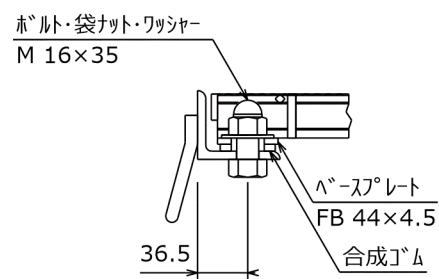
ボルト固定部詳細
