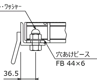
ボルト固定部詳細
