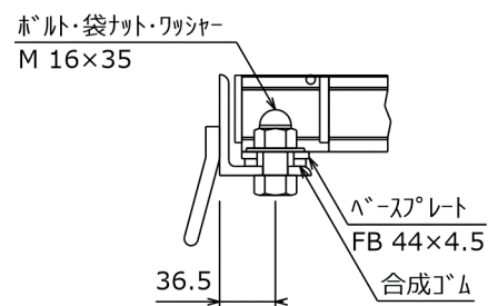
ボルト固定部詳細
