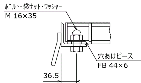
ボルト固定部詳細
