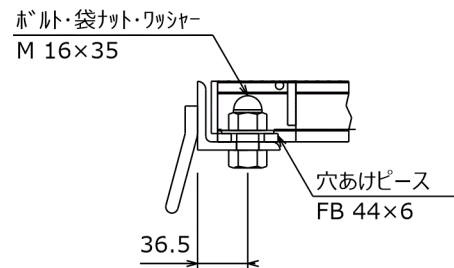
ボルト固定部詳細
