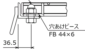
ボルト固定部詳細
