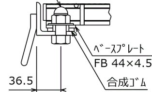
ボルト固定部詳細
