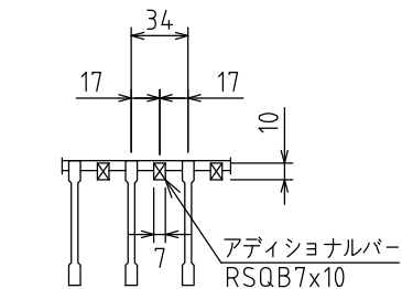
グレーチング詳細図
