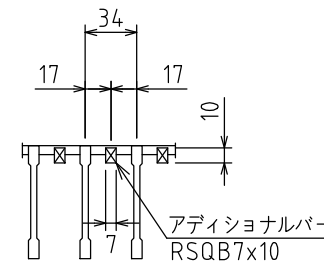
グレーチング詳細図
