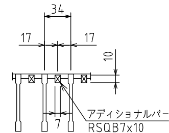
グレーチング詳細図
