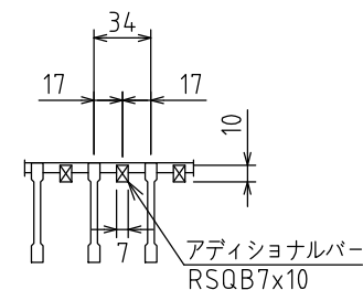
グレーチング詳細図
