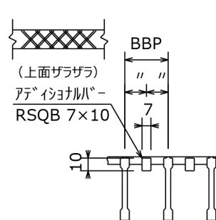
A 矢視断面詳細
