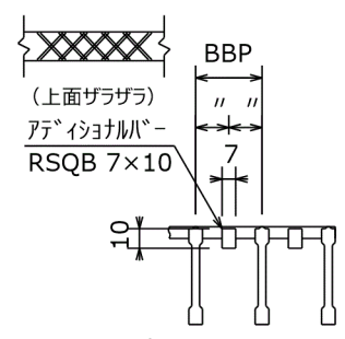
A 矢視断面詳細
