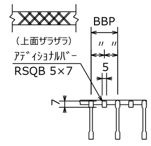
A 矢視断面詳細
