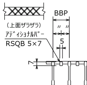
A 矢視断面詳細
