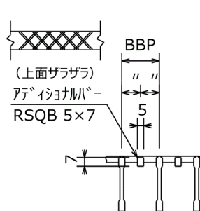
A 矢視断面詳細
