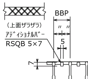
A 矢視断面詳細
