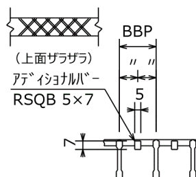
A 矢視断面詳細
