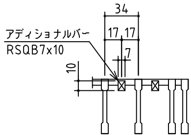
A矢視
