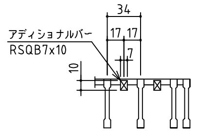
A矢視
