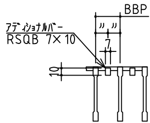
A矢視断面詳細
