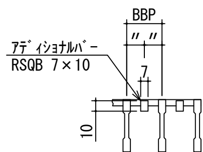
A 矢視断面詳細
