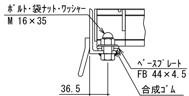
ボルト固定部詳細
