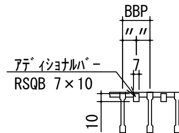
A矢視断面詳細
