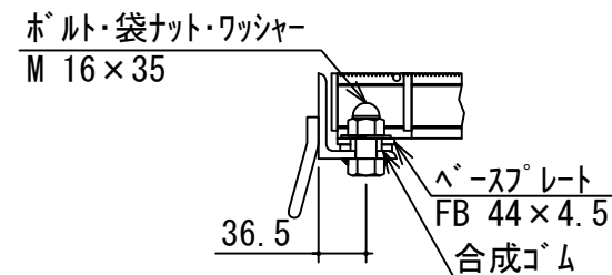
ボルト固定部詳細
