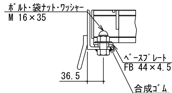
ボルト固定部詳細
