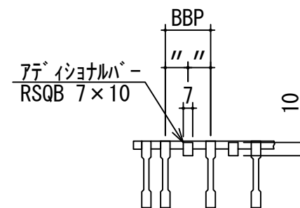
A 矢視断面詳細
