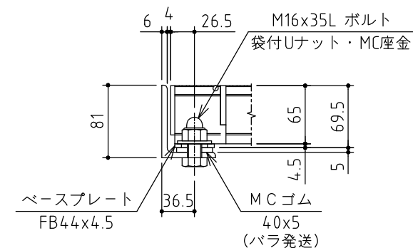
ボルト固定部詳細図 S=1/6
