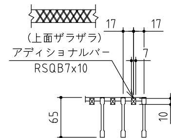
グレーチング断面詳細 S=1/6
