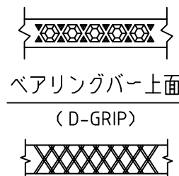
アディショナルバー上面 (ガラガラ)
