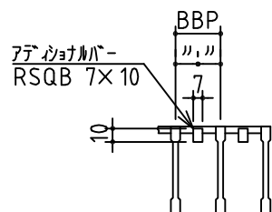
A矢視断面詳細
