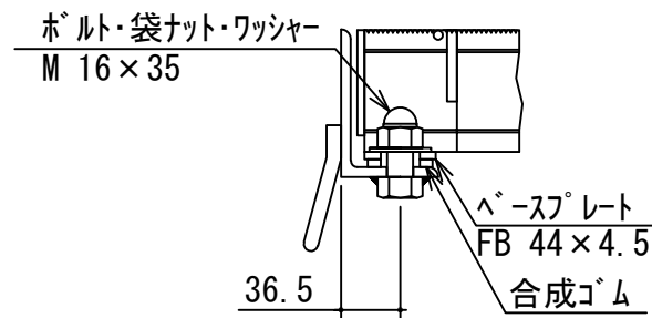
ボルト固定部詳細
