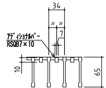
A 矢視断面詳細
