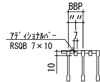
A 矢視断面詳細
