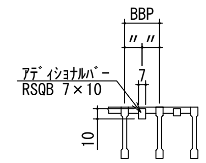
A矢視断面詳細
