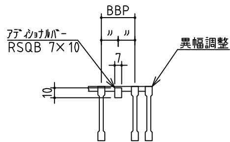
A矢視断面詳細
