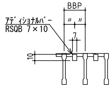
A矢視断面詳細
