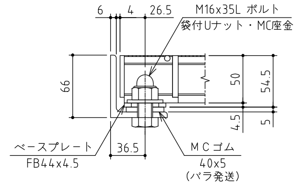
ボルト固定部詳細図
