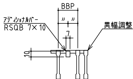
A矢視断面詳細
