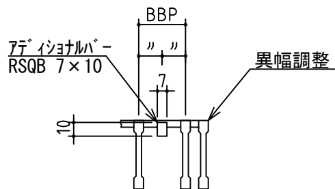
A矢視断面詳細
