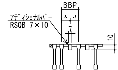
A矢視断面詳細
