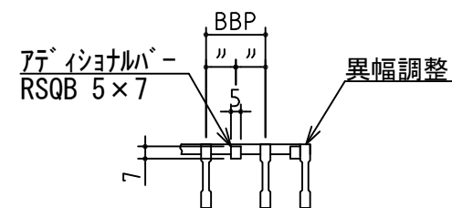
A 矢視断面詳細
