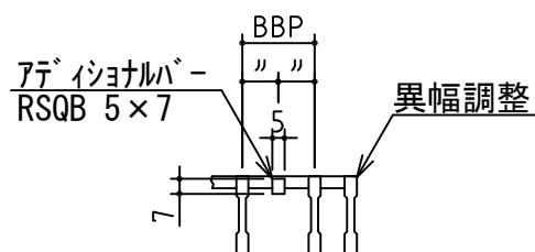
A矢視断面詳細
