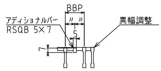
A矢視断面詳細
