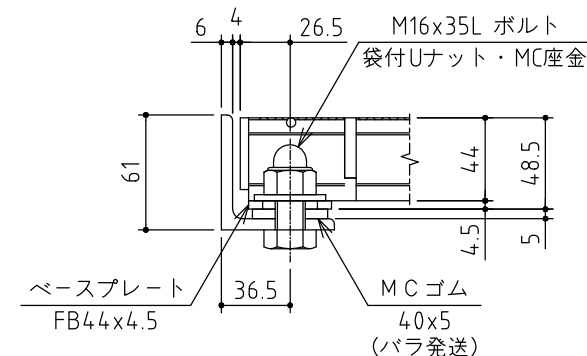
ボルト固定部詳細図 S=1/4
