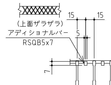
グレーチング断面図
