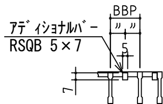
A 矢視断面詳細
